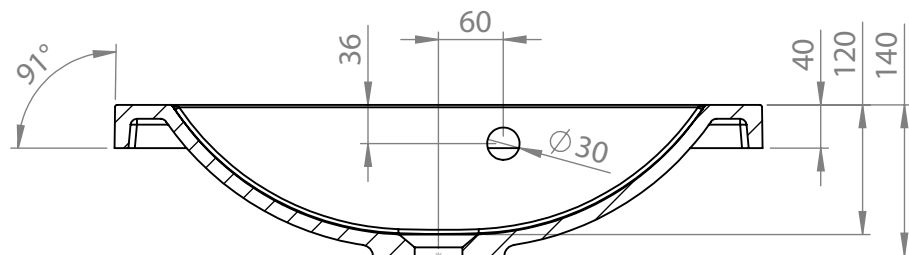
PRZEKRÓJ N-N SKALA 1:7
